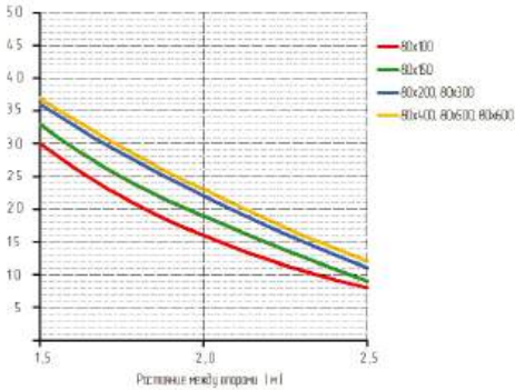
График нагрузки:
