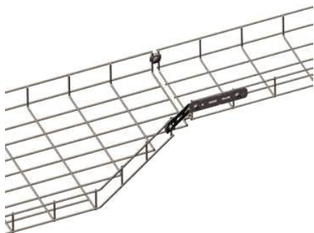
Сужение 1 сторона 60x200-400
