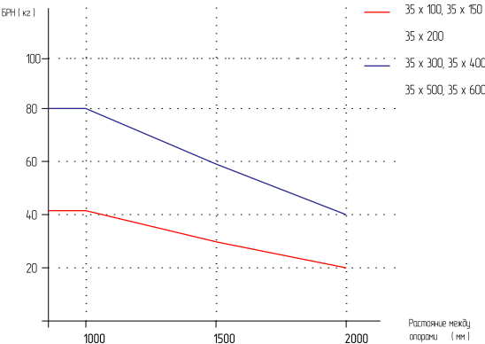
График нагрузки:
