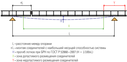
Размещение креплений:
