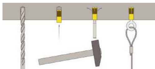
Примеры монтажа
