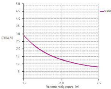
График нагрузки:
