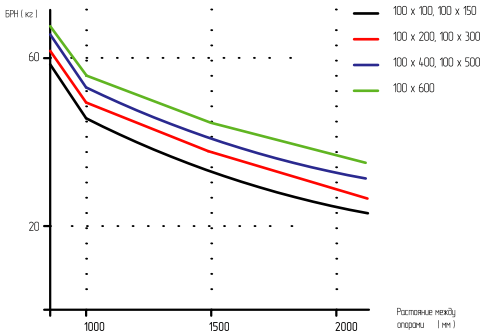
График нагрузки:
