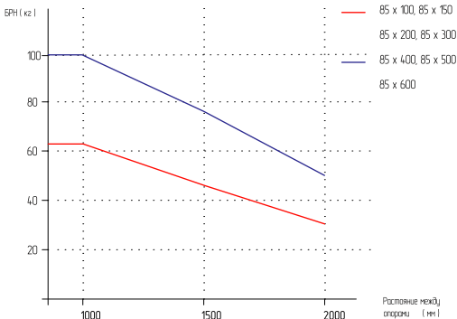
График нагрузки:
