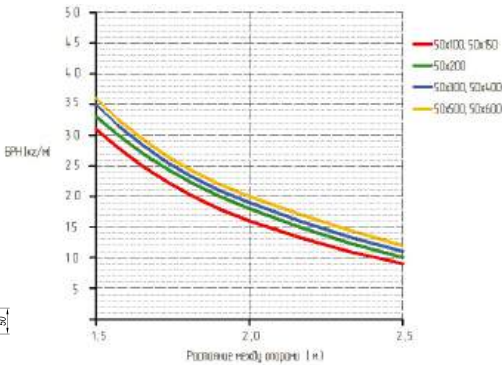
График нагрузки:
