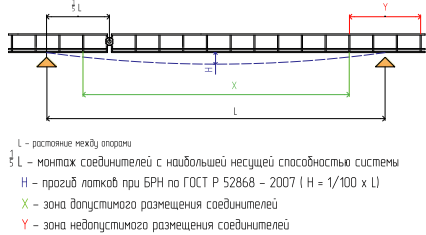
Размещение креплений:
