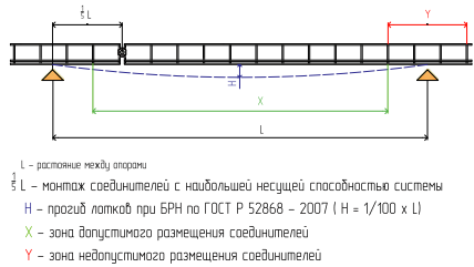
Размещение креплений:
