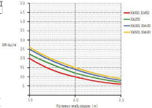
График нагрузки:
