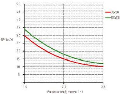
График нагрузки:
