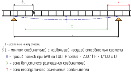
Размещение креплений:
