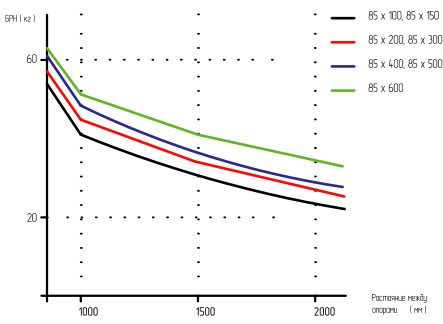
График нагрузки:
