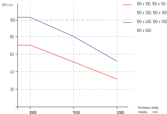
График нагрузки:
