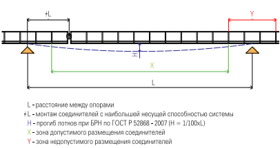
Размещение креплений:
