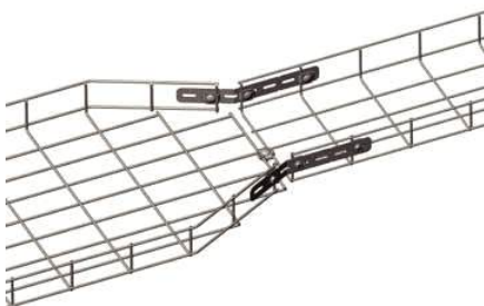
Сужение 2 стороны 60x400-200
